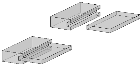
Embrèvement à languette rapportée
