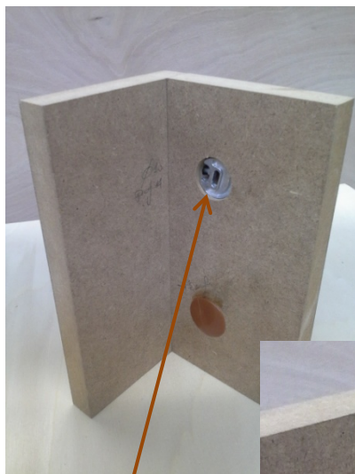
Assemblage par excentrique et goujon
