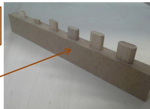
Assemblage par faux tenon
