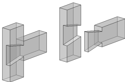
Queue-d'aronde à plat
