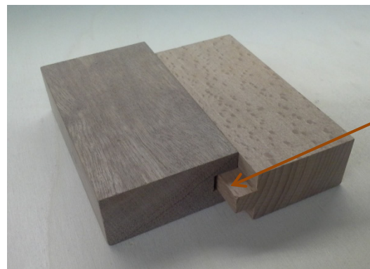
Embrèvement à denture
