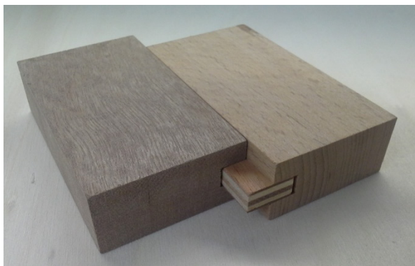
Embrèvement à languette rapportée
