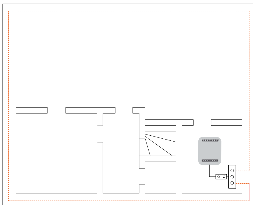
Boucle de terre sous les fondations (min. 60 cm de profondeur)
