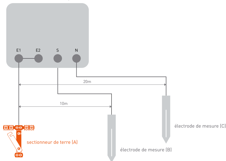
mesure de la résistance de dispersion à la terre
